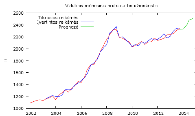
9 pav. Kintamojo W tikrųjų, įvertintų reikšmių bei prognozių grafinis vaizdavimas
