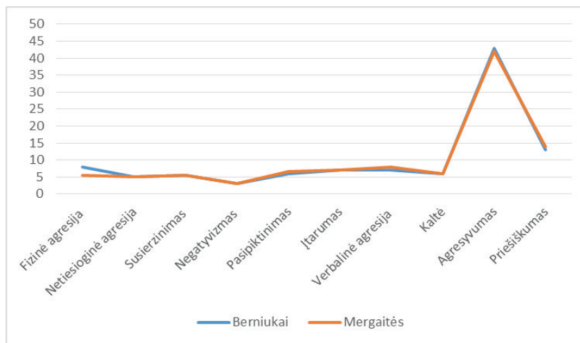
1 pav. Agresyvumo lygio diagnostikos rezultatai, tyrime taikant Bass'o ir Perry'o klausimyną
