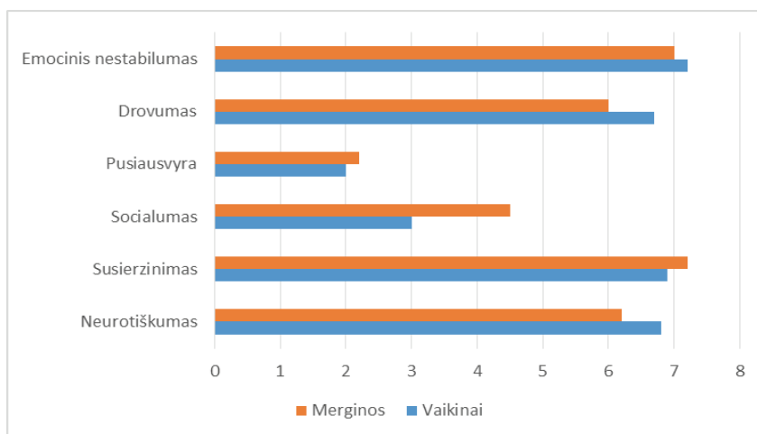
2 pav. Tyrimo rezultatai, gauti taikant modifikuotą Freiburgo asmenybės klasifikaciją (forma B (FPI-B))
