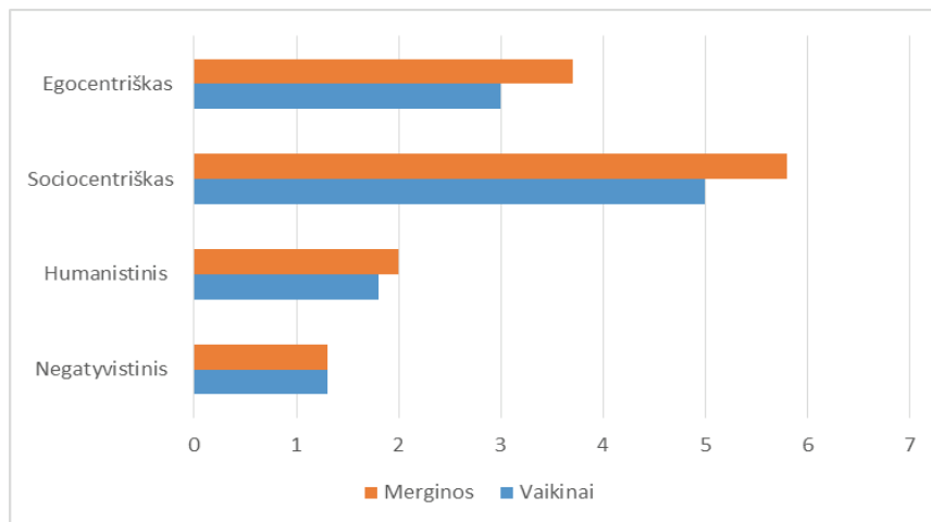
3 pav. Tyrimo rezultatai, gauti taikant Egorychevos technologiją „Asmeninis orientacijos tyrimas“
