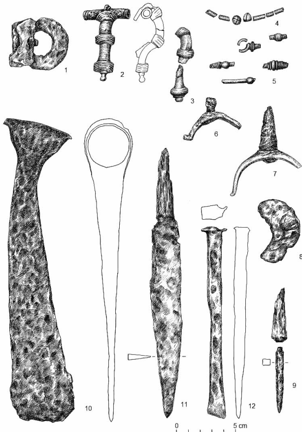
Abb.8. Gräberfeld Mazkatuži, Grab 23, Grabbeiga-ben. 1, 8 – Schnallen, Eisen (A 9952:17, 27); 2–3 – Sprossenfibeln, Bronze (A 9952:11, 12); 4 – Halsring, Bronze (A 9952:8); 5 – Fragmente der Riemenanhänger (?), Bronze (A 9952:13); 6–7 – Sporen, Bronze, Eisen (A 9952:21, 22); 9 – Priem, Eisen (A 9952:18); 10 – Schmalaxt, Eisen (A 9952:1); 11 – Dolch, Eisen (A 9952:9); 12 – Meißel, Eisen (A 9952:10). Zeichnung Dz. Zemīte.
