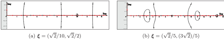
Fig. 3. Domain \mathcal{N} for \xi_1/\xi_2 = m/n \in \mathbb{Q} , \xi_1, \xi_2 \notin \mathbb{Q} .
